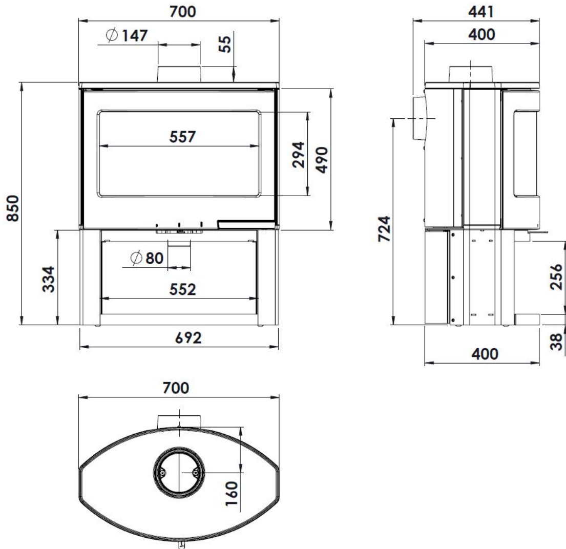
Abbildung Nr.1 - Abmessungen des Geräts in mm Tarbes-Dublin
