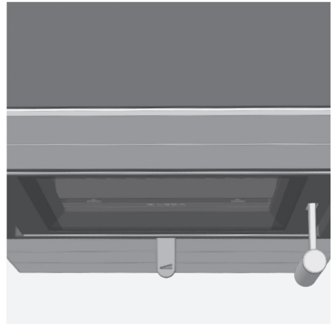
Abb. 4.9 Verbrennungslufthebel mittig, Verbrennungsluft auf Nennwärmeleistung
